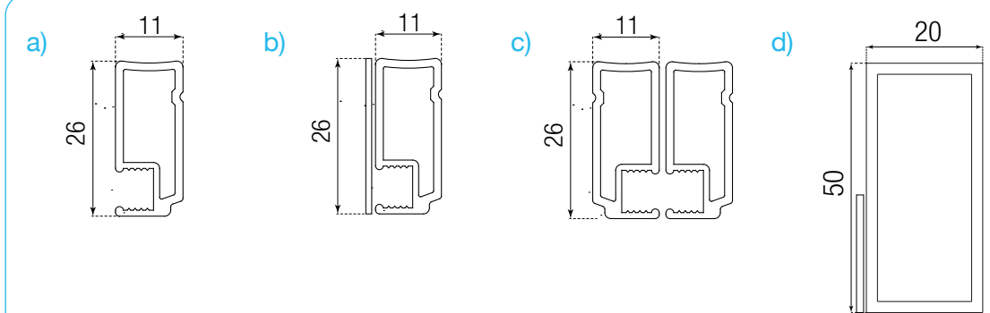
a) POMPEI SINGOLA (profilo 26x11 singolo)
