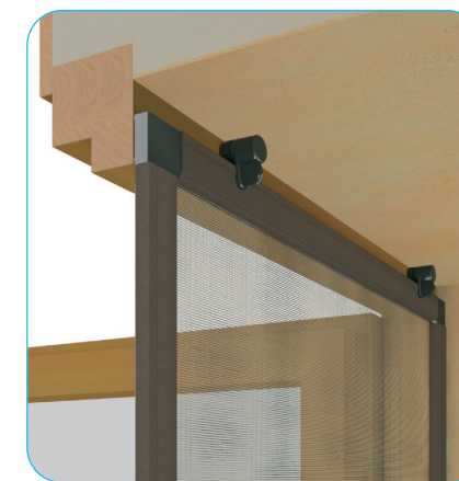
Applicazione attacchi di fissaggio "a coccinella"
