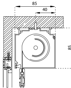
Montaggio a soffitto/parete diretto Top/front fix without bracket
